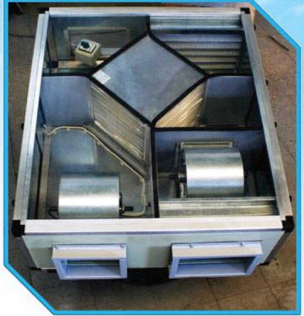
ISI GERİ KAZANIM CİHAZI
